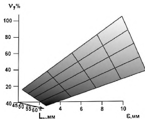
Рис. 2. Залежність рівномірності розподілу насіння по ширині захвату сошника V від довжини похилої ділянки – L_H і ексцентриситету установки ділянки – \varepsilon . розподільник у вигляді тіла обертання (варіант1)
